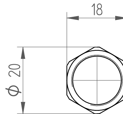
Befestigungsmutter Mounting nut
