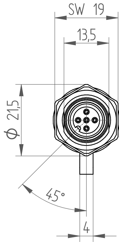
Lochbild Hole pattern
