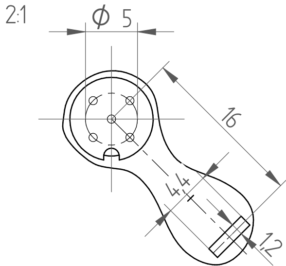
Lochbild Hole pattern
