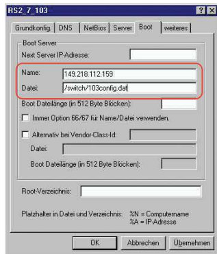
Abb. 62: Konfigurationsdatei auf dem tftp-Server
