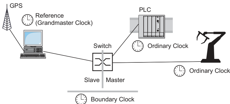
Abb. 19: Position der Boundary-Clock in einem Netz
