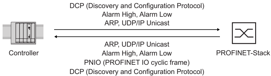
Abb. 54: Kommunikation zwischen Controller und dem Gerät
