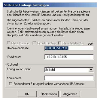
Abb. 66: Einträge für statische Adressen
