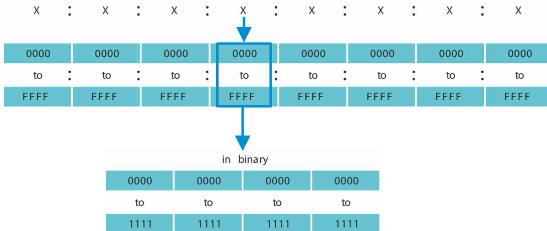
Abb. 12: Darstellung der IPv6-Adresse
