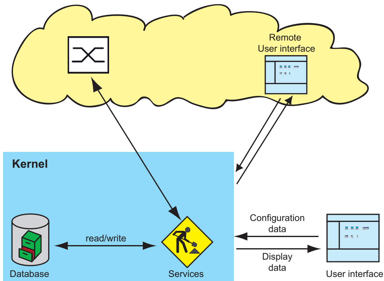
Figura 114:Arquitectura del kernel de Industrial HiVision
